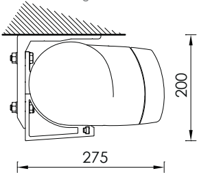
Montaggio a soffitto con terminale a cassonetto * Ceiling installation with box front bar *
