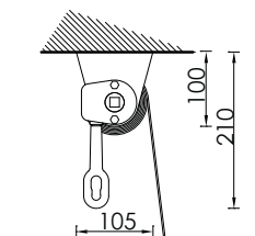
Ingombri senza cassonetto Encumbrance without cassette
