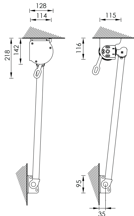
Montaggio a soffitto Ceiling installation
