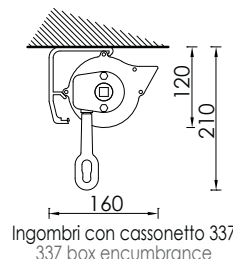
Ingombri con cassonetto 337 337 box encumbrance
