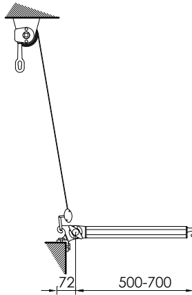
Ingombri con cassonetto 337 337 box encumbrance
