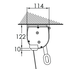
Ingombri con cassonetto FN0941 FN 0941 box encumbrance
