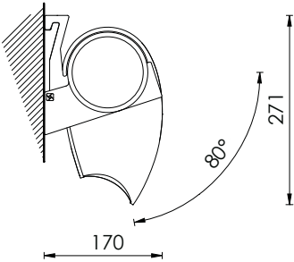
Dimensioni massime - Maxi dimensions
