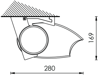
Montaggio a soffitto Ceiling installation
