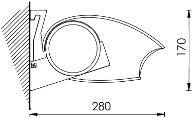
Montaggio a parete 80° Wall installation 80°
