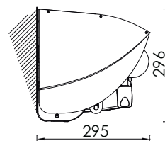
Montaggio con tettuccio Installation with a hood
