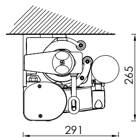
Montaggio a soffitto Ceiling installation
