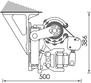
Montaggio a soffitto Ceiling installation
